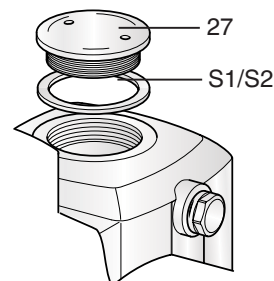
рис. М-2: Демонтаж запорной пробки
