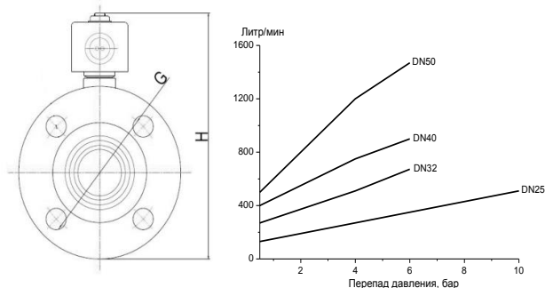
Диаграмма 1. Зависимость расхода от давления
