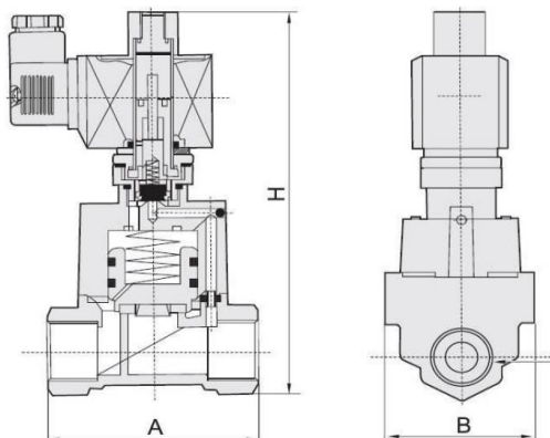
Рисунок 1. Эскиз
