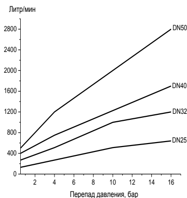
Диаграмма 1. Зависимость расхода от давления
