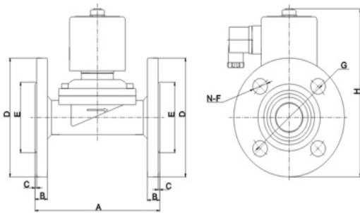
Рисунок 1. Эскиз
