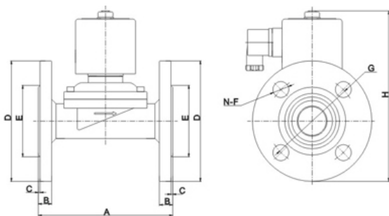
Рисунок 1. Эскиз
