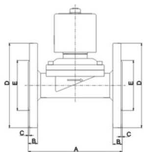
Рисунок 1. Эскиз
