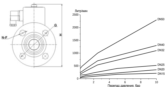
Диаграмма 1. Зависимость расхода от давления
