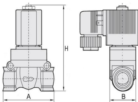
Рисунок 1. Эскиз
