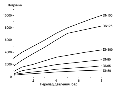
Диаграмма 1. Зависимость расхода от давления
