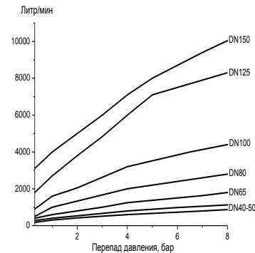
Диаграмма 1. Зависимость расхода от давления
