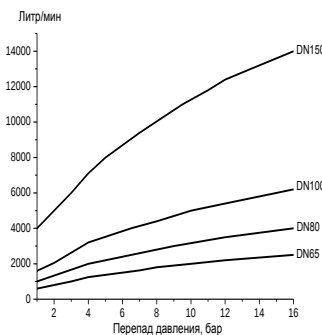
Диаграмма 1. Зависимость расхода от давления
