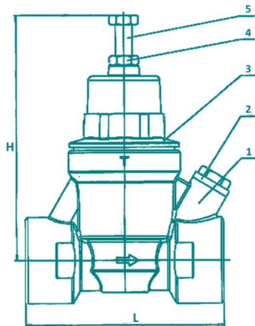
Рисунок 1. Эскиз
