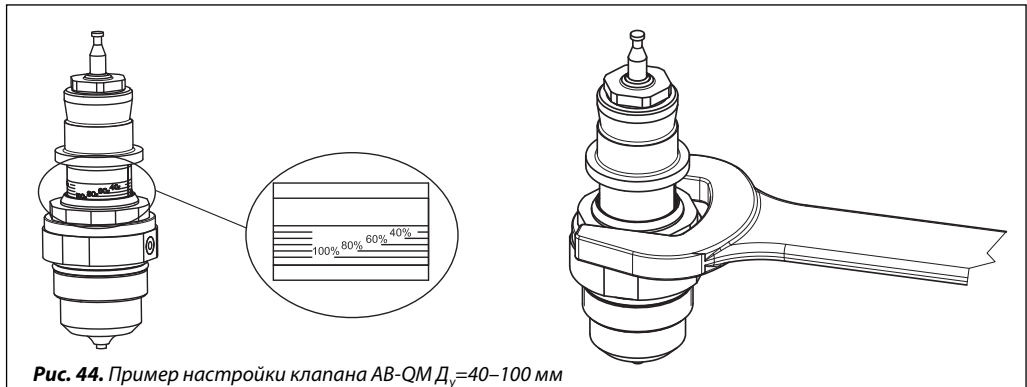
Рис. 44. Пример настройки клапана АВ-QM D_y=40-100 мм
