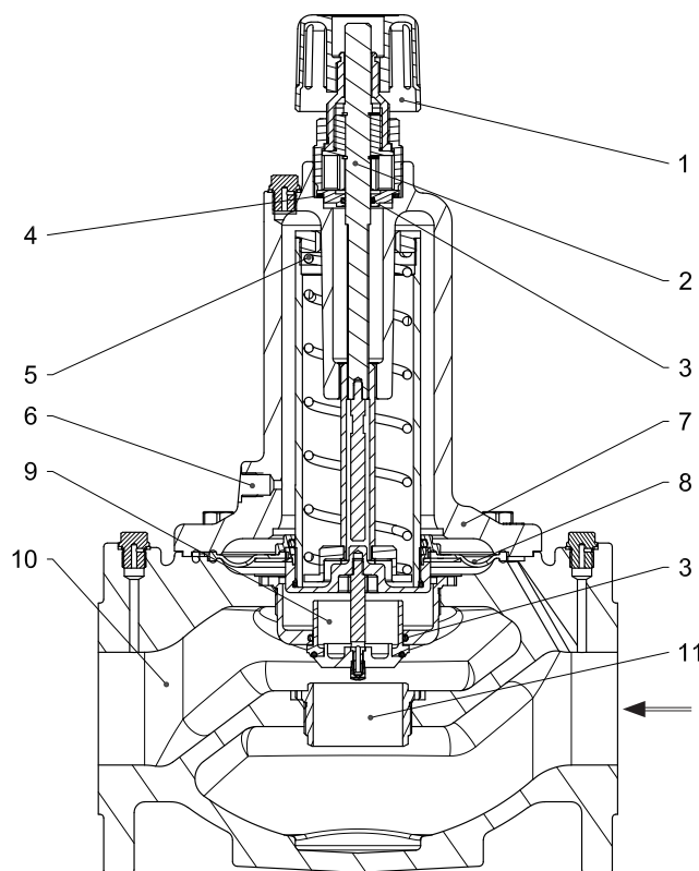
Рис. 11. ASV-PV Д у = 65–100 мм
