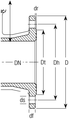
Drillings to ISO 7005 part 2 (EN 1092-2: 1997, DIN 2501):
