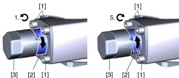
рис. 15: концевой упор
