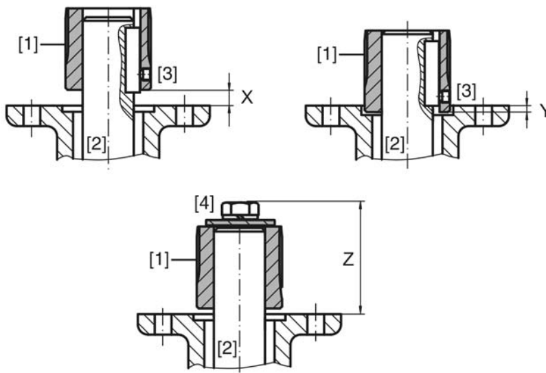
рис. 5: Установочные размеры муфты
